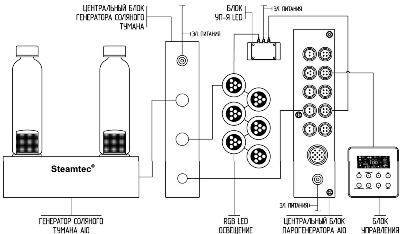
Рисунок 4: Центральный блок генератора соляного тумана Работа с моделью АЮ
