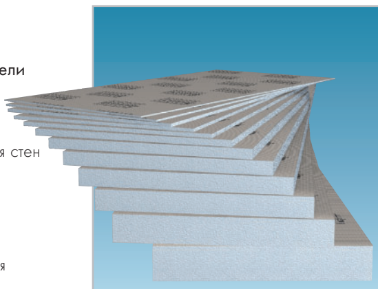
ELEMENT-EL – универсальная конструкционная панель для прикручивания к деревянным и металлическим каркасам, ...
